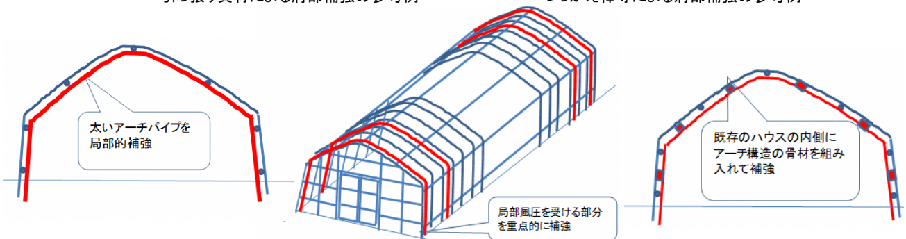
太めのパイプにて局部的に補強の参考例
